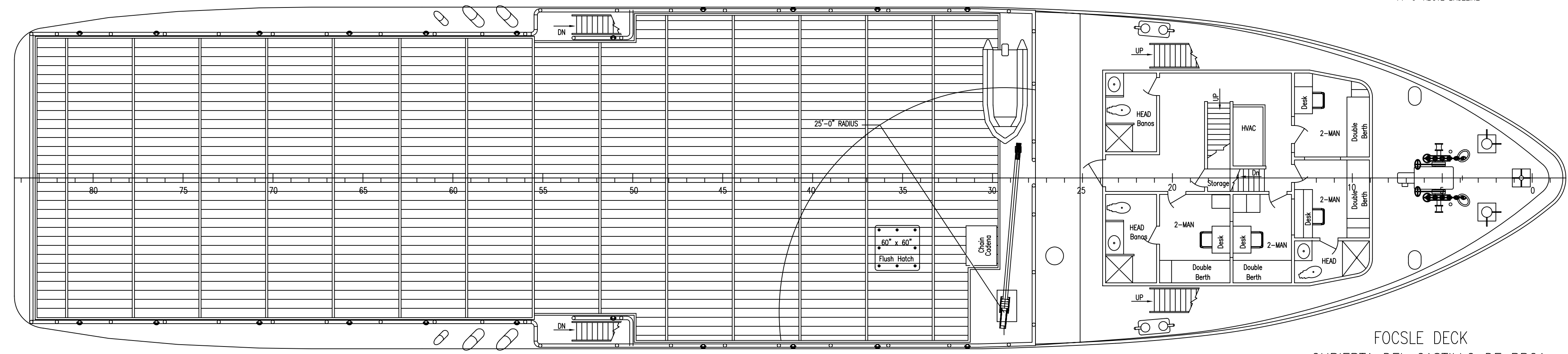
FOCSLE DECK CUBIERTA DEL CASTILLO DE PROA 24'-0" ABOVE BASELINE
