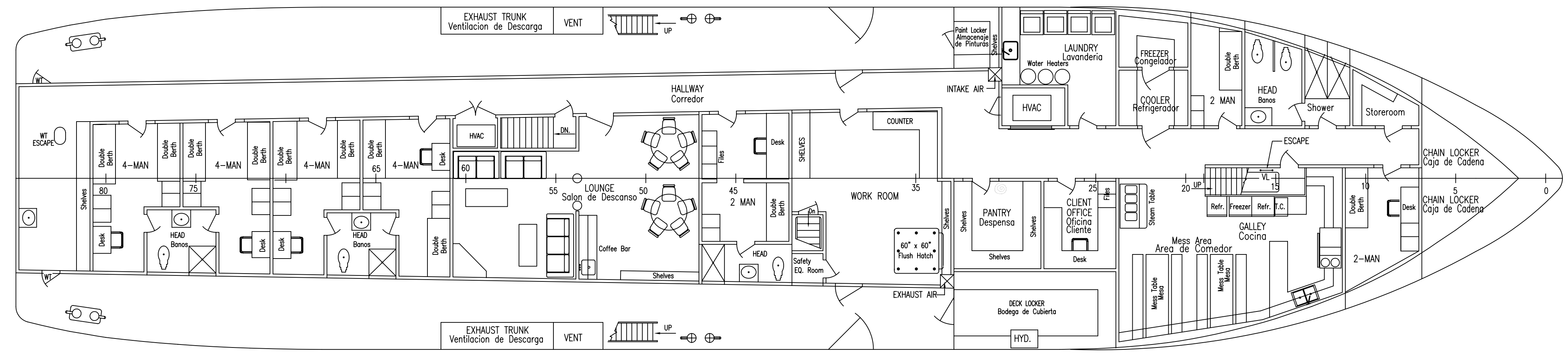
MAIN DECK PLAN DE CUBIERTA PRINCIPAL 14'-0" ABOVE BASELINE
