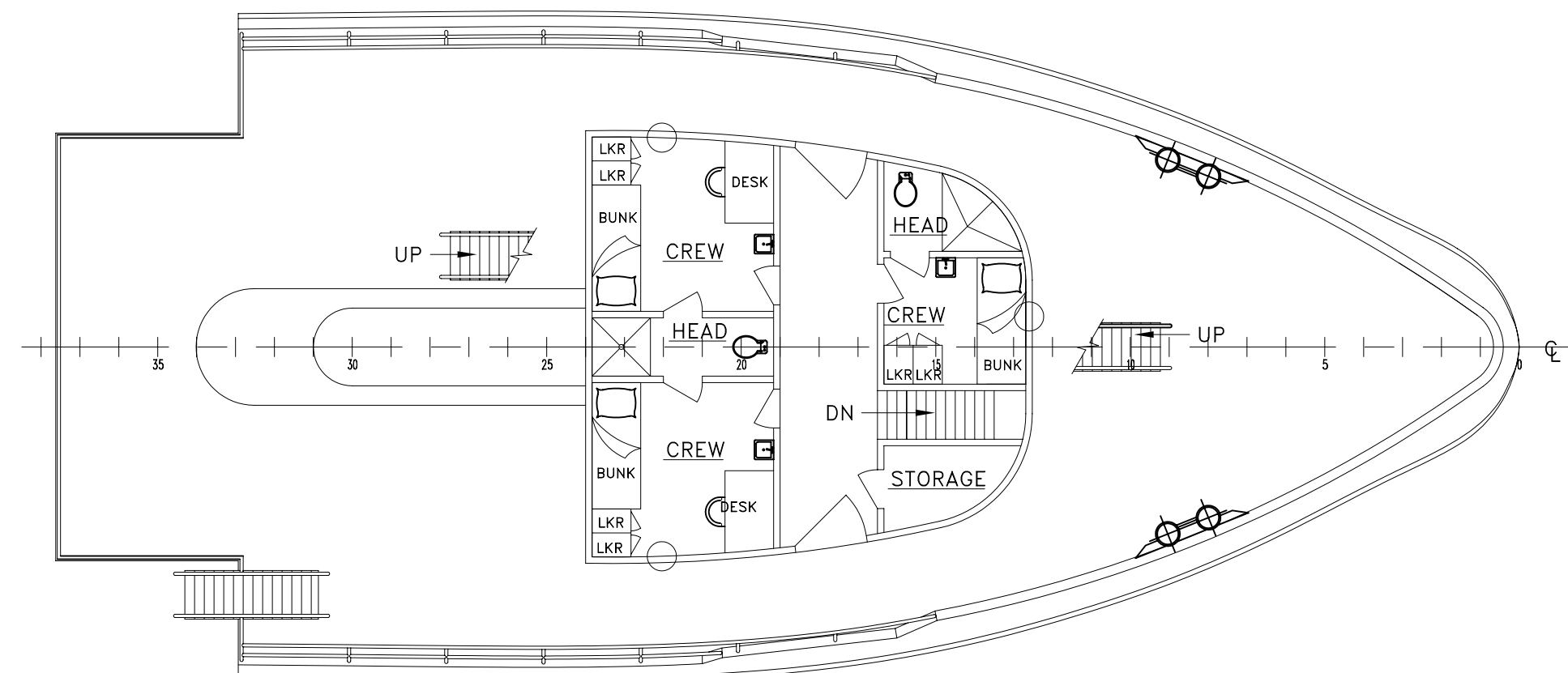
FOCSLE DECK SCALE: 1/8"=1'-0"
