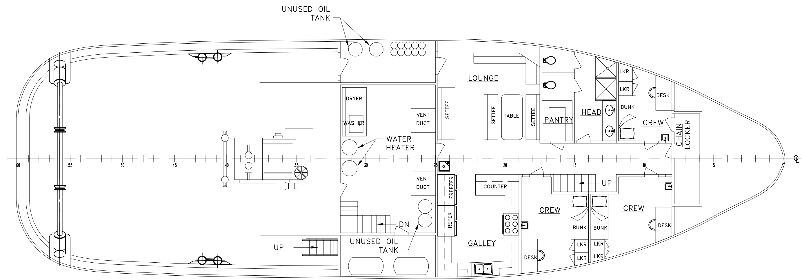
MAIN DECK SCALE: 1/8"=1'-0"
