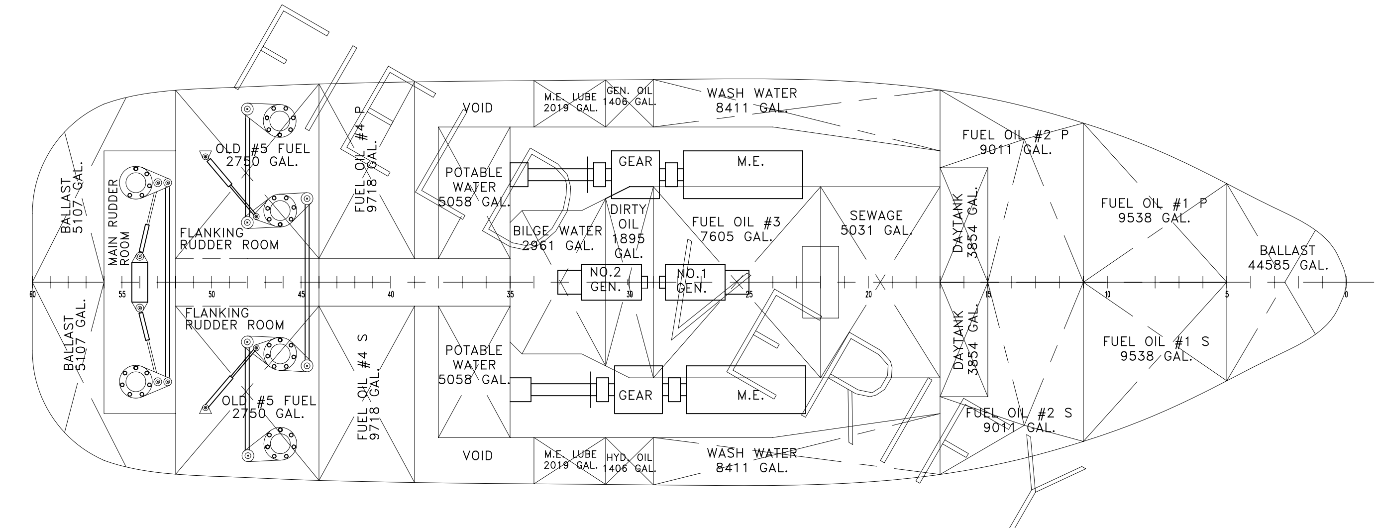
HOLD PLAN SCALE: 1/8"=1'-0"
